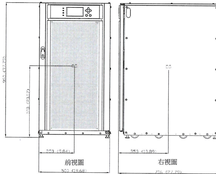
圖 3-5: UPS 機櫃的重心位置(93ET 20kVA)
