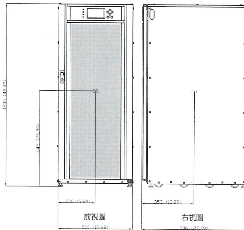
圖 3-6: UPS 機櫃的重心位置(93ET 30kVA)
